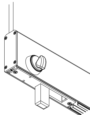
Verrou de plancher à 1 barillet à clé et 1 bouton activé en façades.
