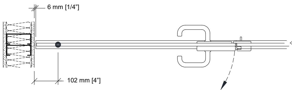
6 Optional pivot door
