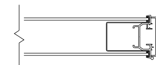
6 End cap
