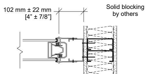
5 Wall jamb (optional)
