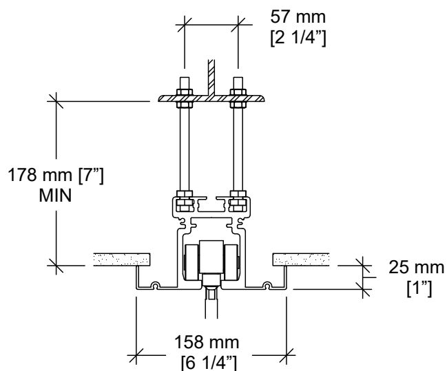
Rail d'aluminium #55-T (Chariot #53)
