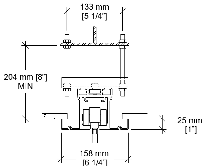
Rail d'aluminium #55-T (Chariot #53) et support de rail optionnel
