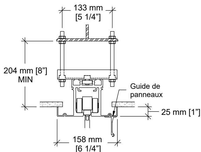
Rail #55-T (Chariot #53) et support de rail optionnel
