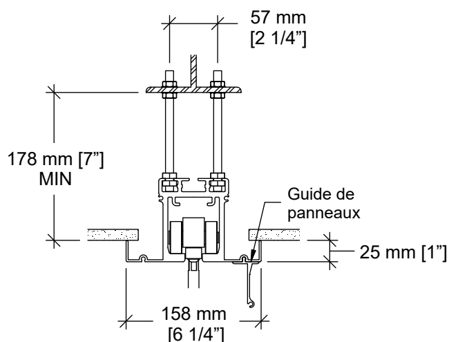
Rail d'aluminium #55-T (Chariot #53)
