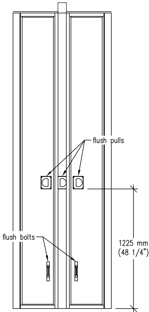
Elevation
