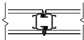
⑧ Joint de panneaux sans moulures verticales apparentes (optionnel) (CTS 49 et plus)
